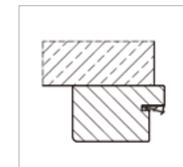
Blendrahmen
