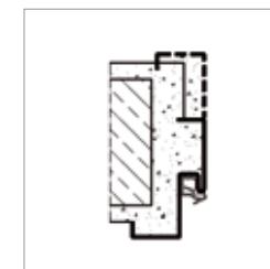
Stahlumfassungszarge
