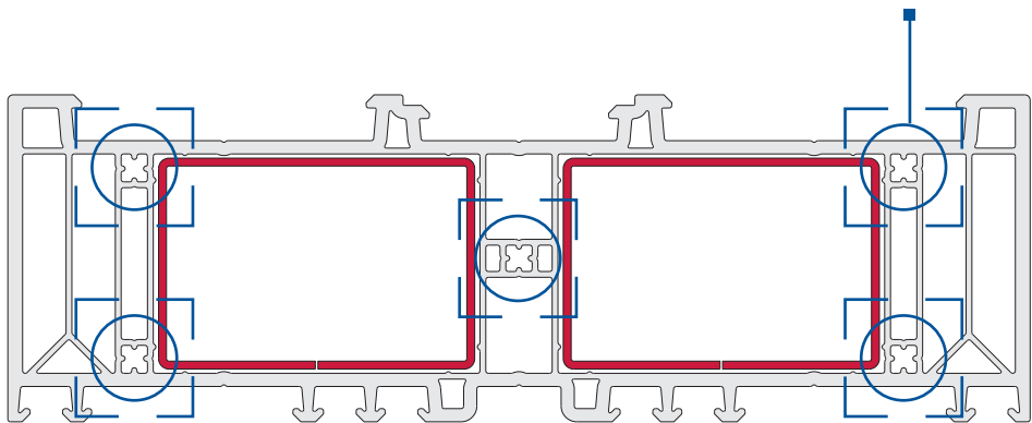
Integrierte Schraubkanäle Fünf integrierte Schraubkanäle sorgen für eine sichere Verschraubung der Zarge. Eine Verschraubung im Stahl ist nicht mehr erforderlich.
