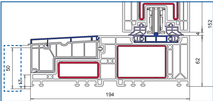
Bauwerksabdichtung: einfach und sicher VEKAMOTION 82 erleichtert die Umsetzung aller Vorgaben zur Bauwerksabdichtung, sodass u. a. die Vorgaben der Schweizer Flachdachrichtlinie problemlos erfüllt werden können. Nach außen bietet das System eine 50 mm hohe, durchgehende PVC-Fläche für eine sichere Abdichtung mit Dichtbahnen bzw. Flüssigabdichtung. Ein zusätzlicher Wetterschenkel oder Steckdeckel ist leicht montierbar.
