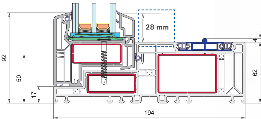
Innenansichtshöhe des Festflügels: 28 mm
